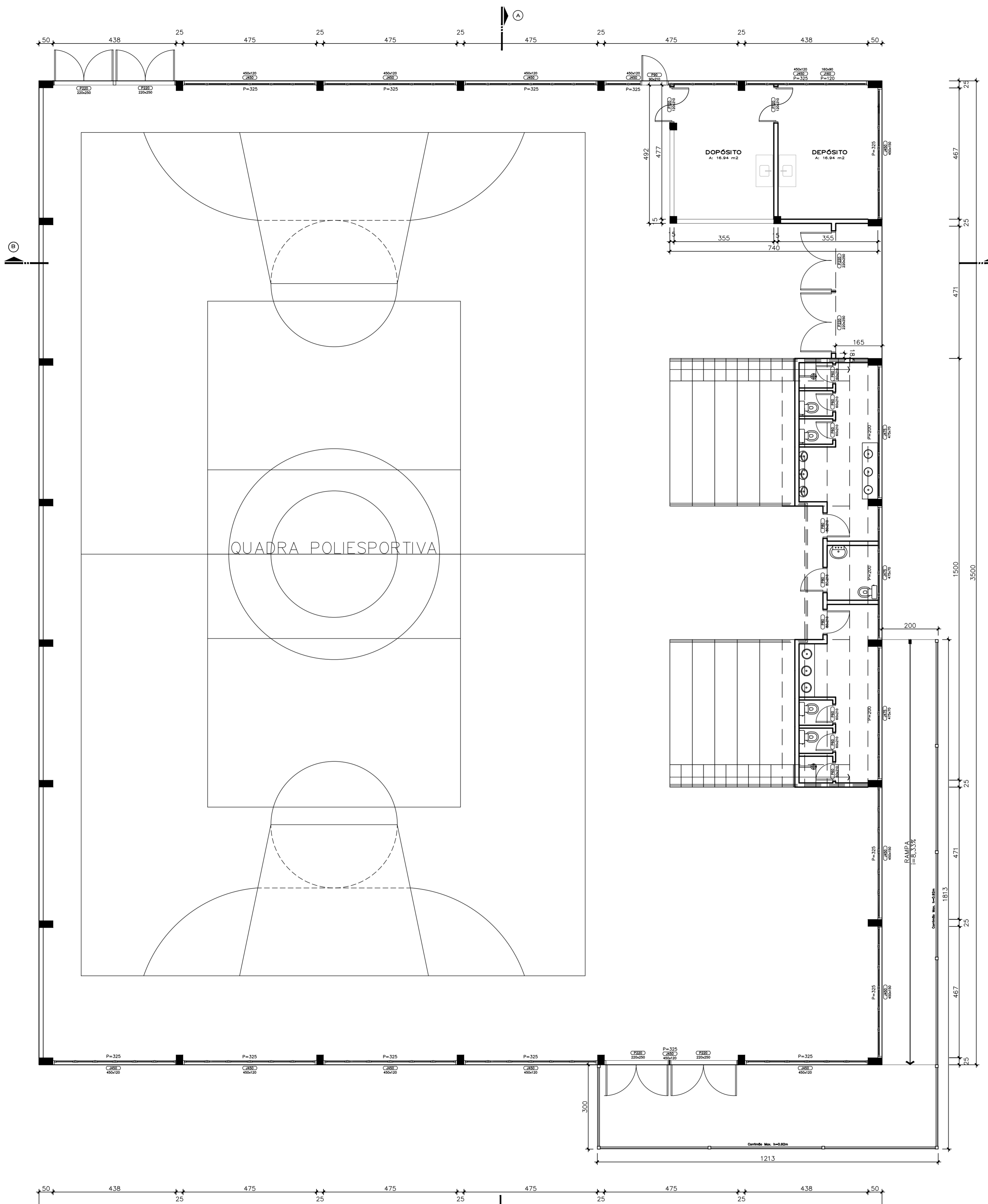
PLANTA BAIXA ÁREA TOTAL A: 1.050,00 m 2
