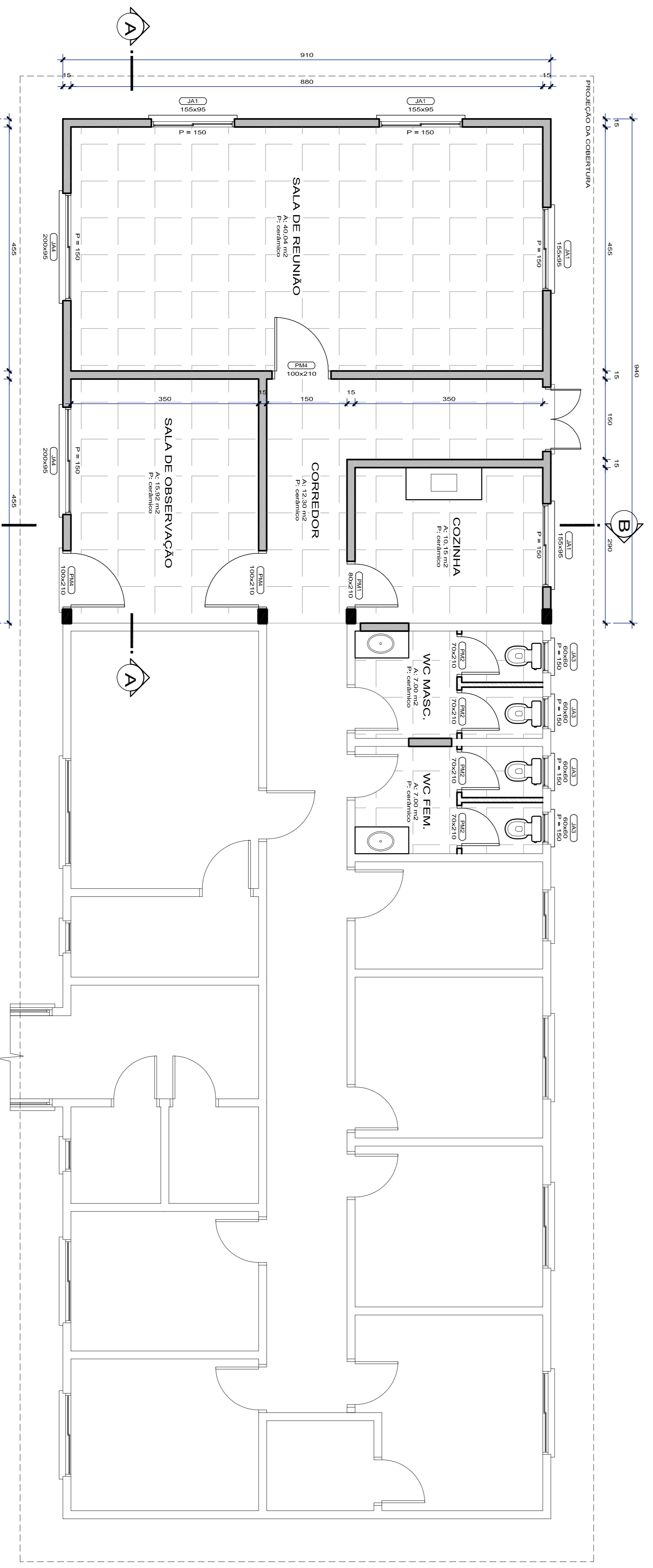
PLANTA BAIXA AMPLIAÇÃO A: 85,54 m 2 ESCALA: 1/50
